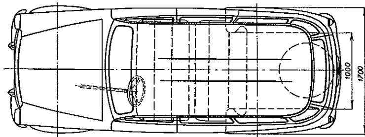
Rozměrový náčrtek vozu STW
